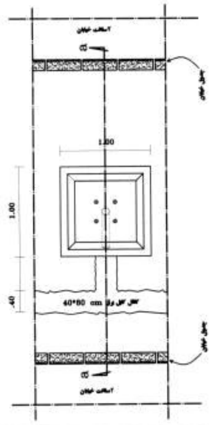
هکابل اندازه گذاری و اجرایی فنداسیون پایه های روشنی (امتری)
