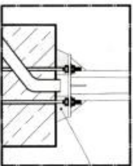
شکل اندازه گذاری و اجرایی فلنسون پایه های روشنی ۹ متری
