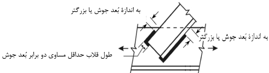
شکل ۶-۹-۲-۱۰ جوش گوشه در انتهای اعضای محوری
